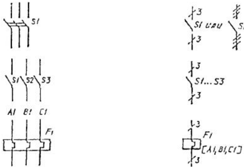
a - многолинейное изображение; б - однолинейное изображение.
